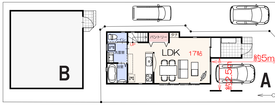
配置イメージ図兼1階平面図 / S1:150
