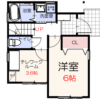
1階平面図 / S1:150
