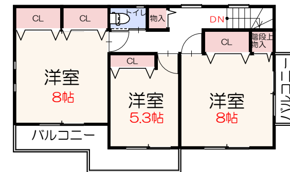
2階平面図 / S1:150
