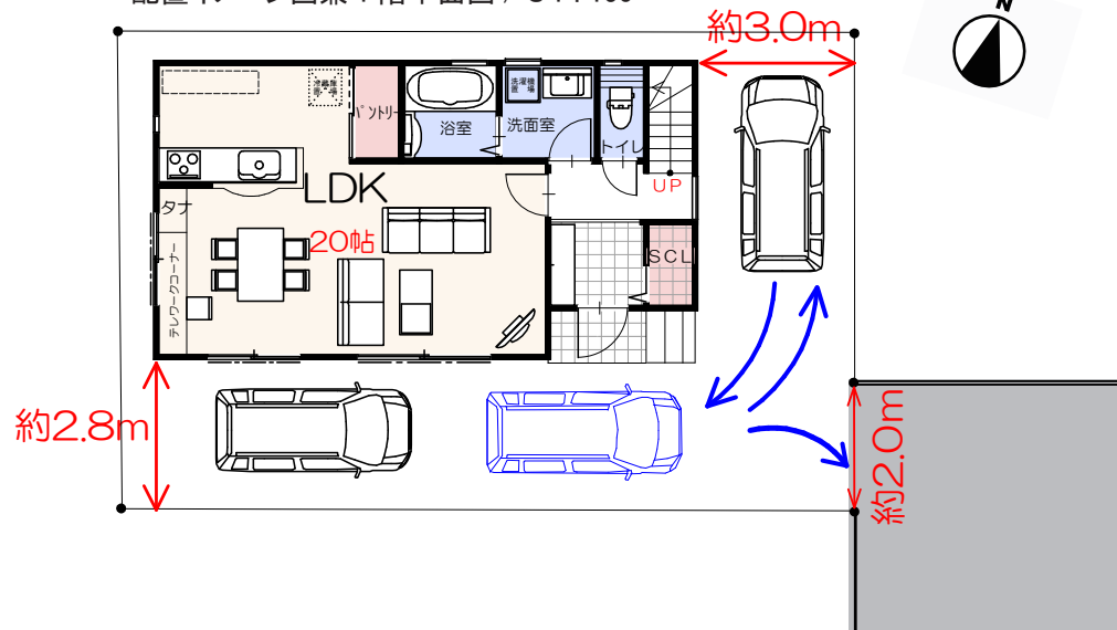
配置イメージ図兼 1階平面図 / S1:150
