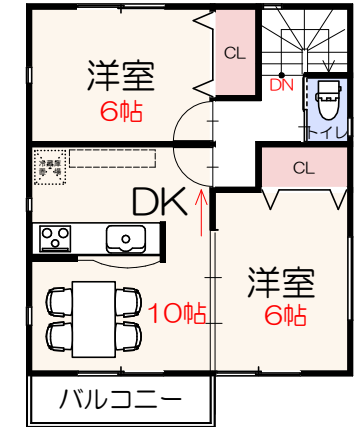
2階平面図 / S1:150
