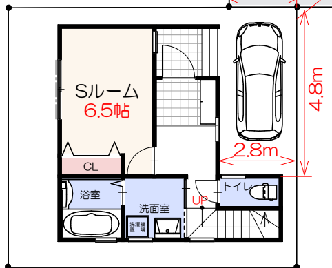
配置イメージ図 兼1階平面図 / S1:150
