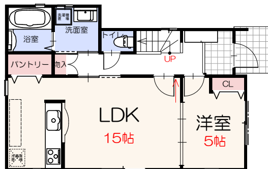
1階平面図 / S1:150
