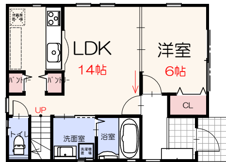
1階平面図 / S1:150
